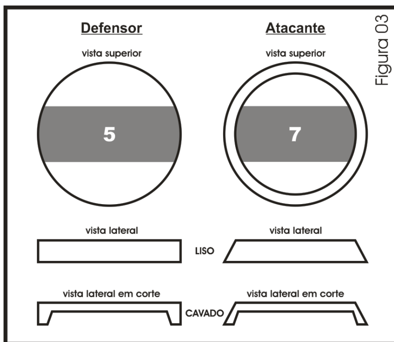
Figura 3 – Os botões: suas formas e medidas máximas.
