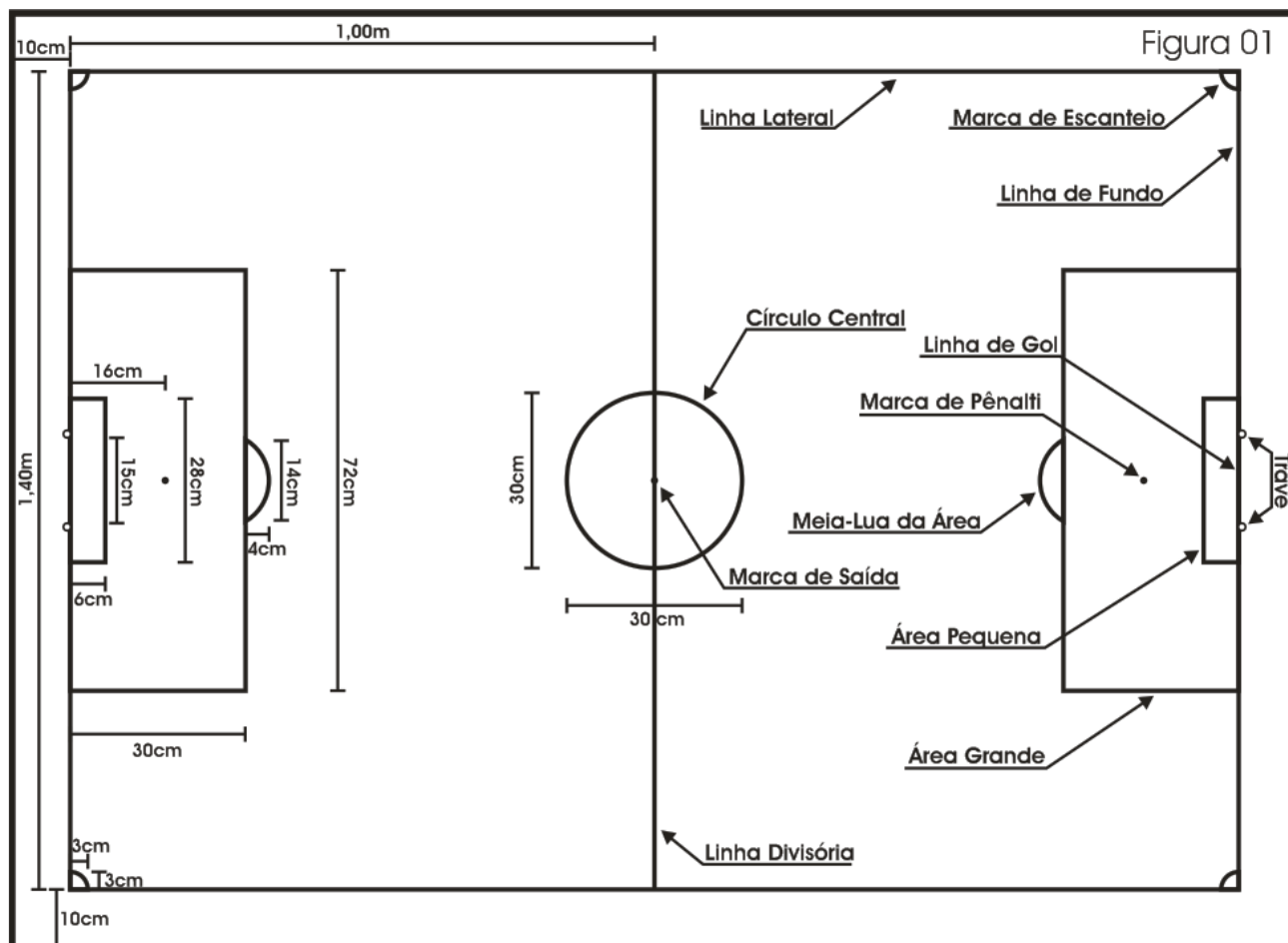
Figura 1 – O campo de jogo: suas marcações e medidas.
