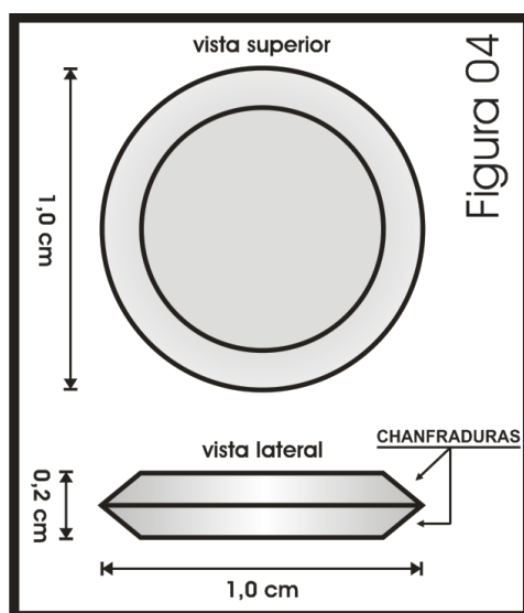
Figura 4 – A bola: seu formato característico e suas medidas.
